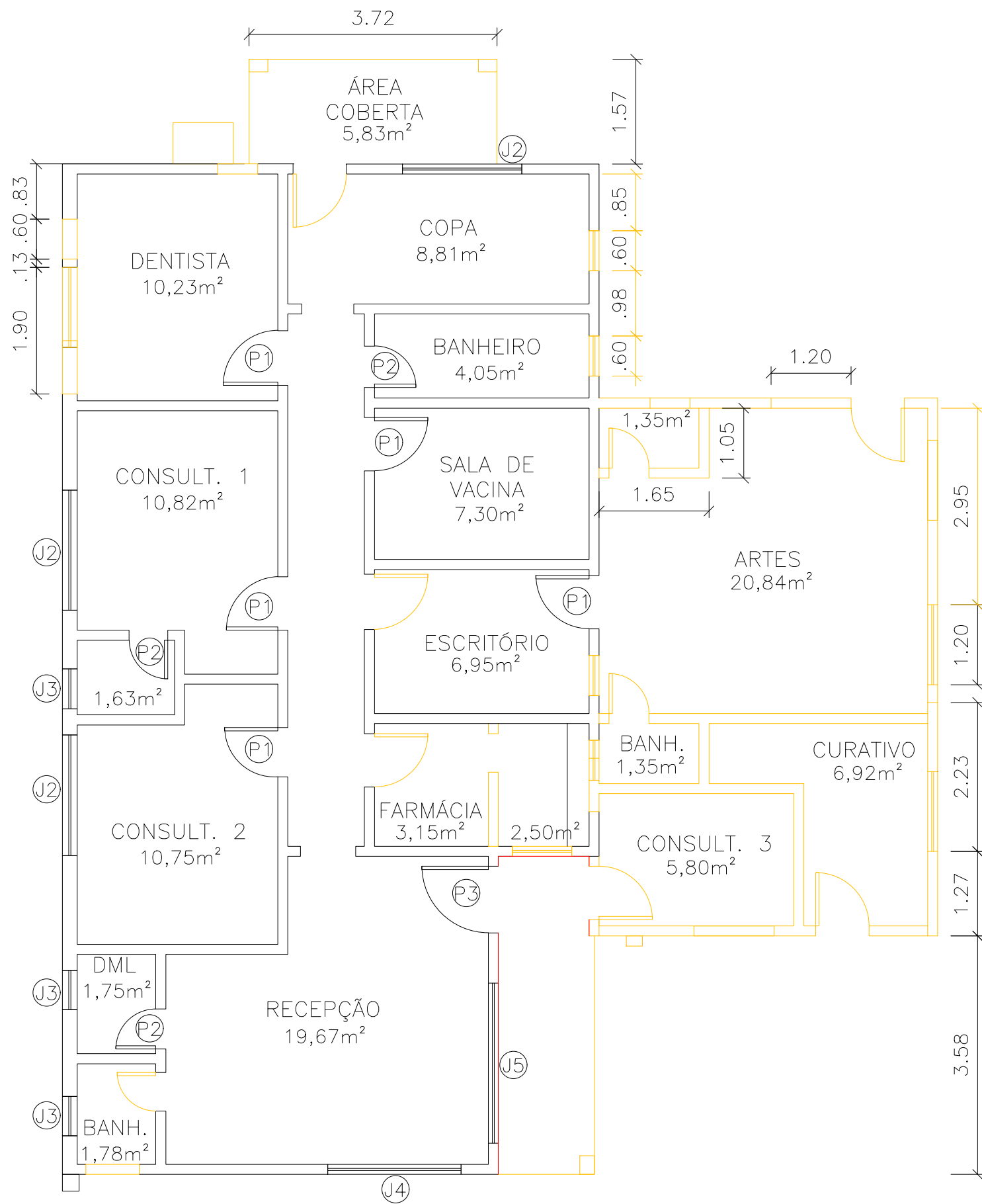
1 PLANTA DE DEMOLIR ESCALA 1:75
