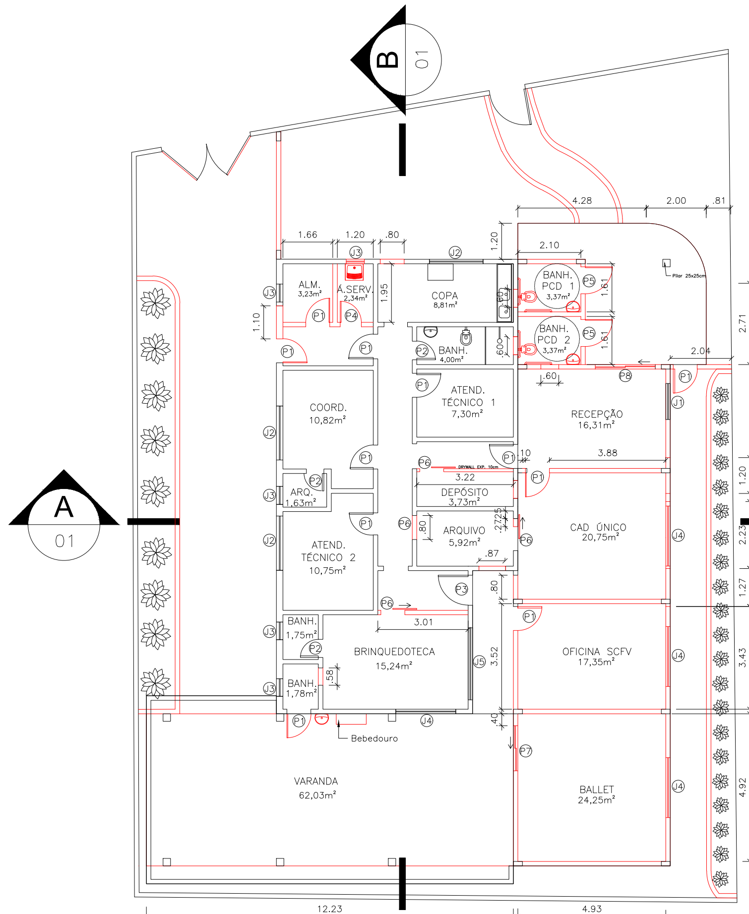
1 PLANTA DE CONSTRUIR ESCALA 1:125
