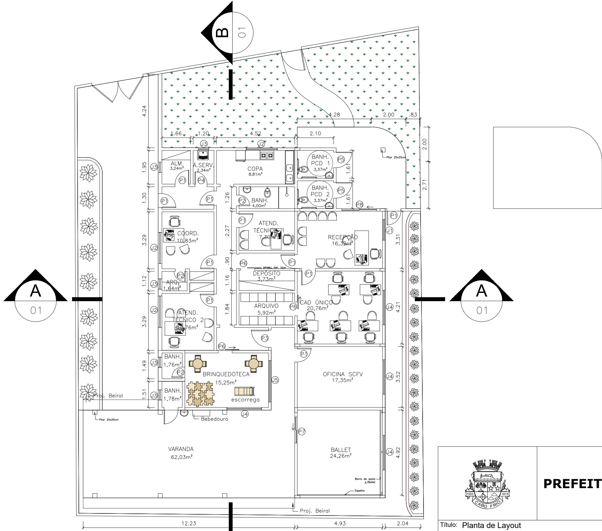
1 PLANTA DE LAYOUT ESCALA 1:130
