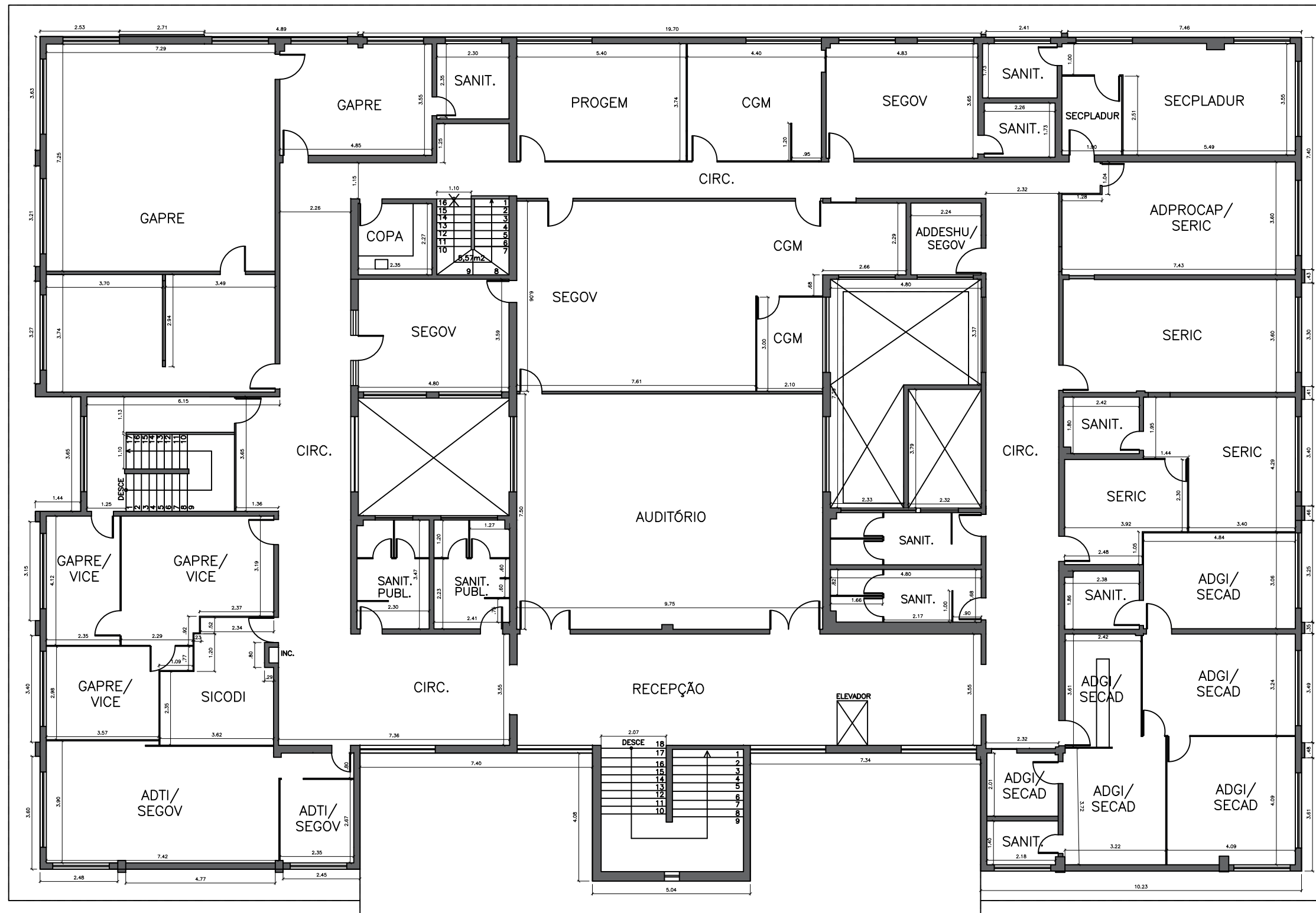
1 PLANTA DO SEGUNDO PAVIMENTO ESCALA 1:125
