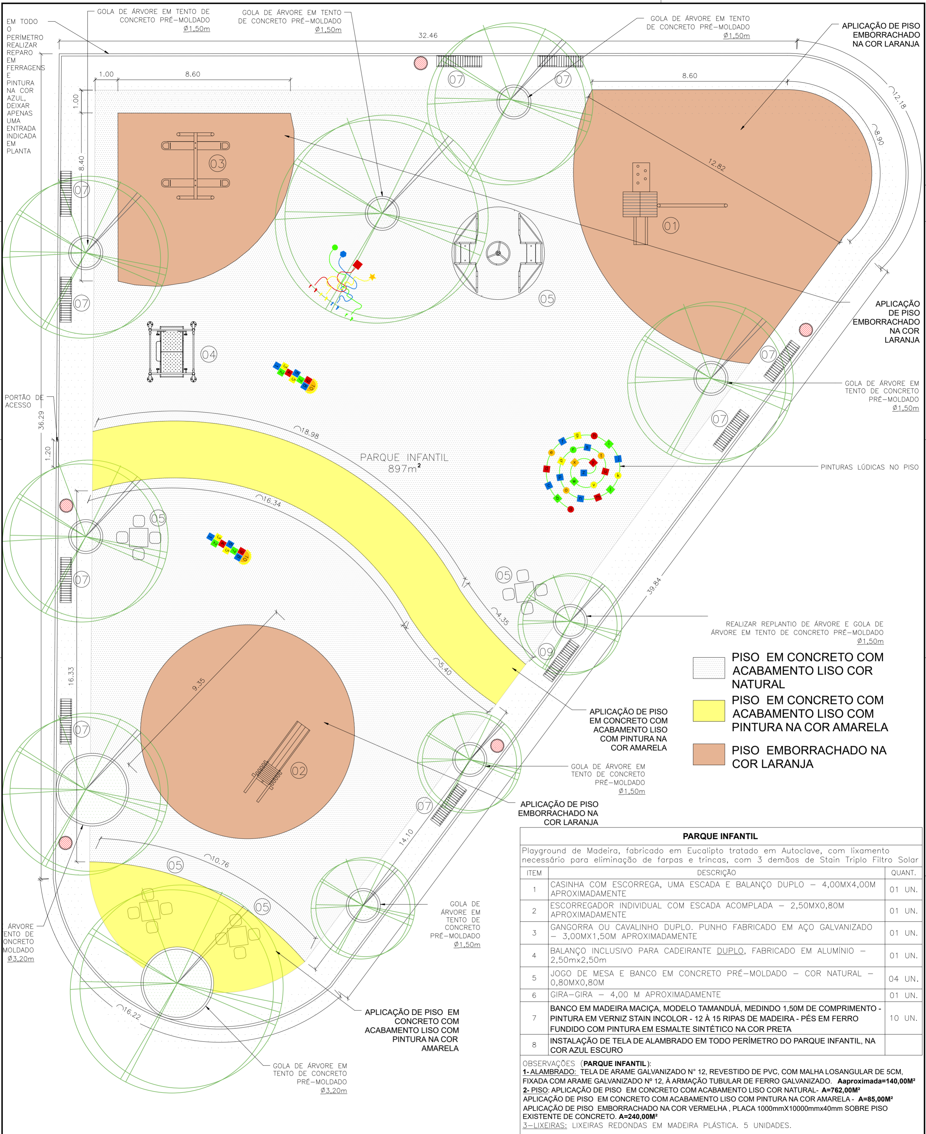
01 PLANTA BAIXA | PARQUE INFANTIL ESCALA 1:100
