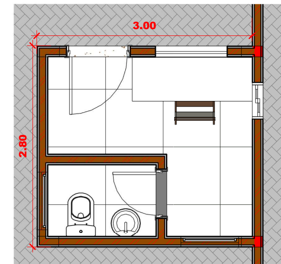
2 Planta de Layout - Térreo 1 : 50
