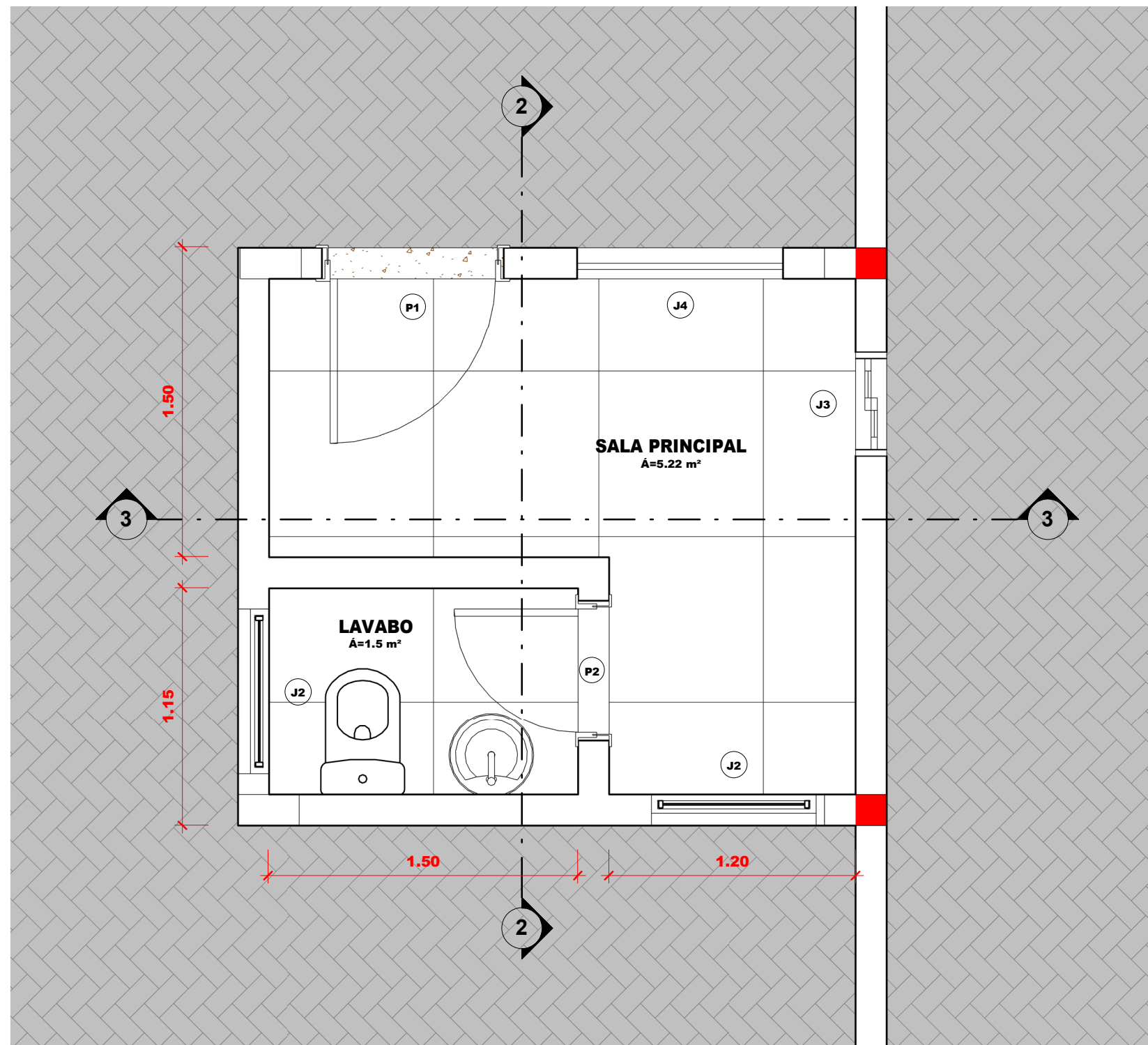
1 Planta de Cota - Térreo 1 : 25
