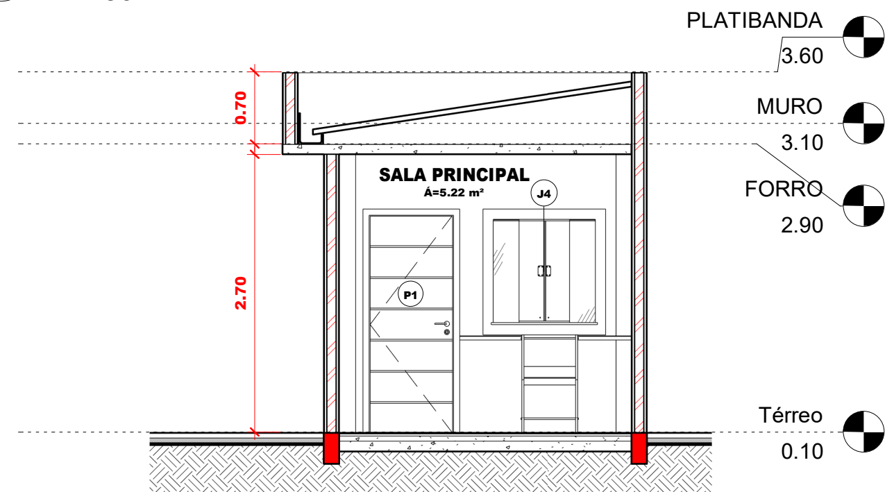
3 Corte Transversal 1 : 50
