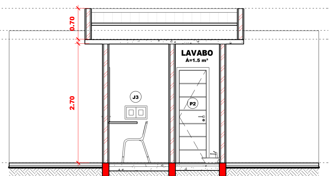
2 Corte Longitudinal 1 : 50
