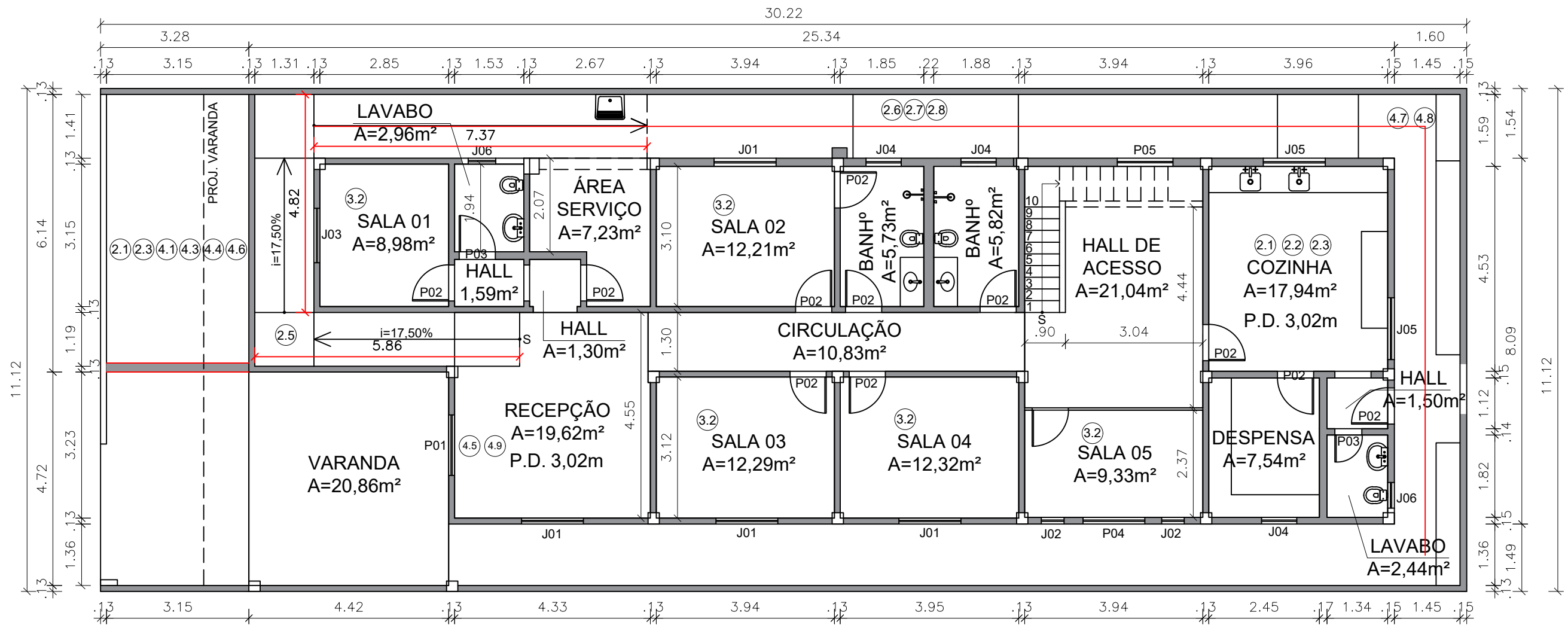
1 PLANTA BAIXA - TÉRREO ESCALA 1:100
