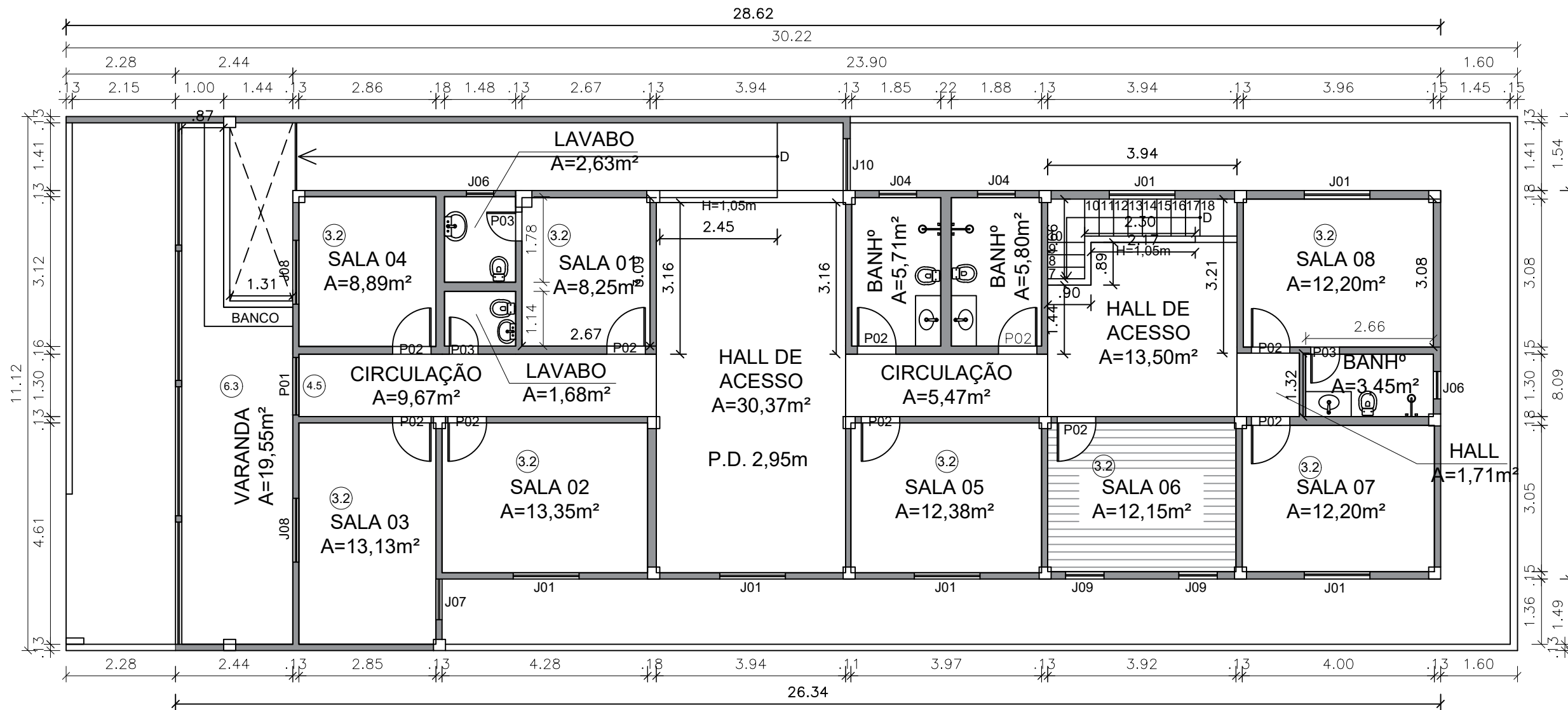
1 PLANTA BAIXA - 1º PAVIMENTO ESCALA 1:100
