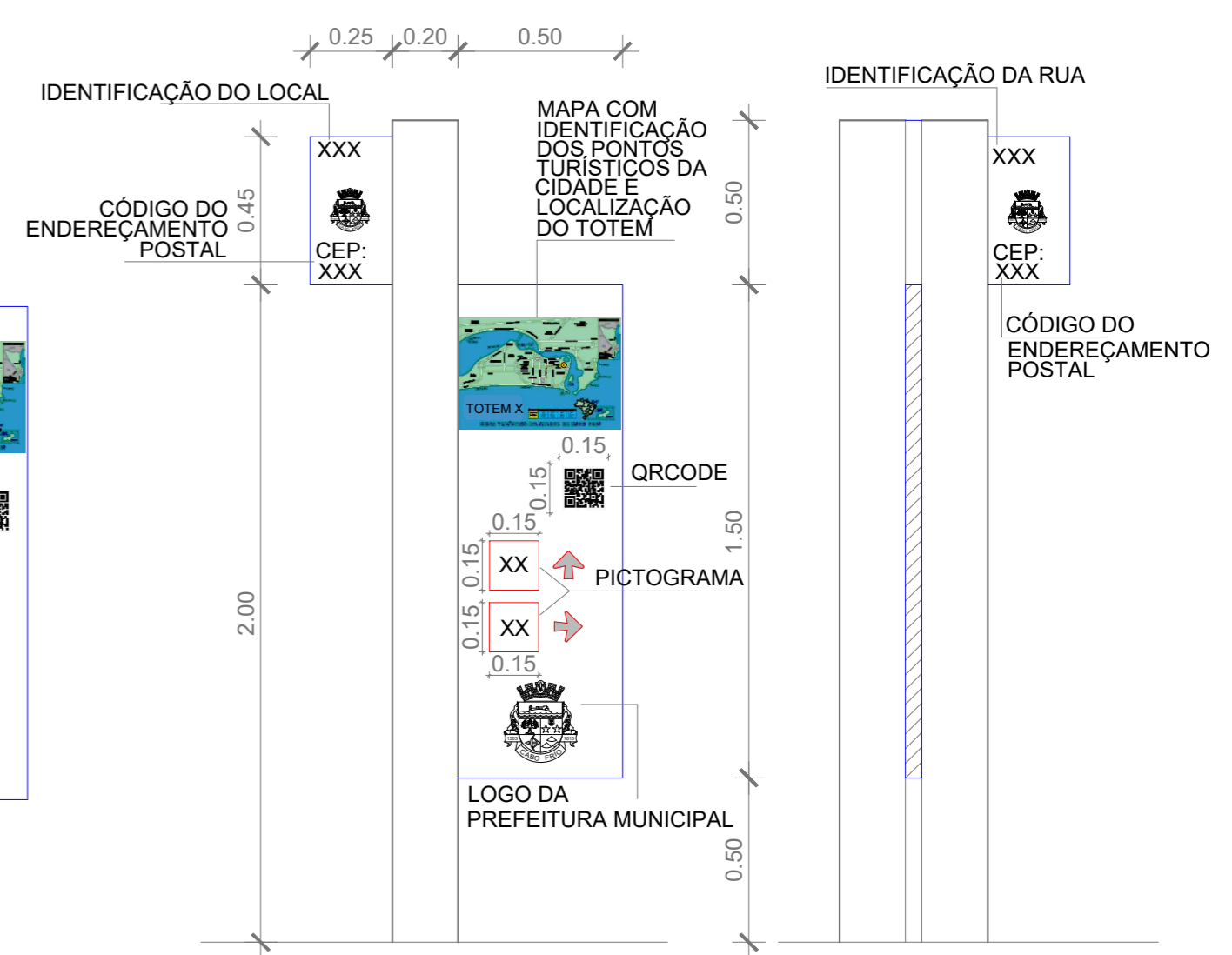
TOTENS DE SINALIZAÇÃO TURÍSTICA - DETALHE TÍPICO ESCALA - 1:20
