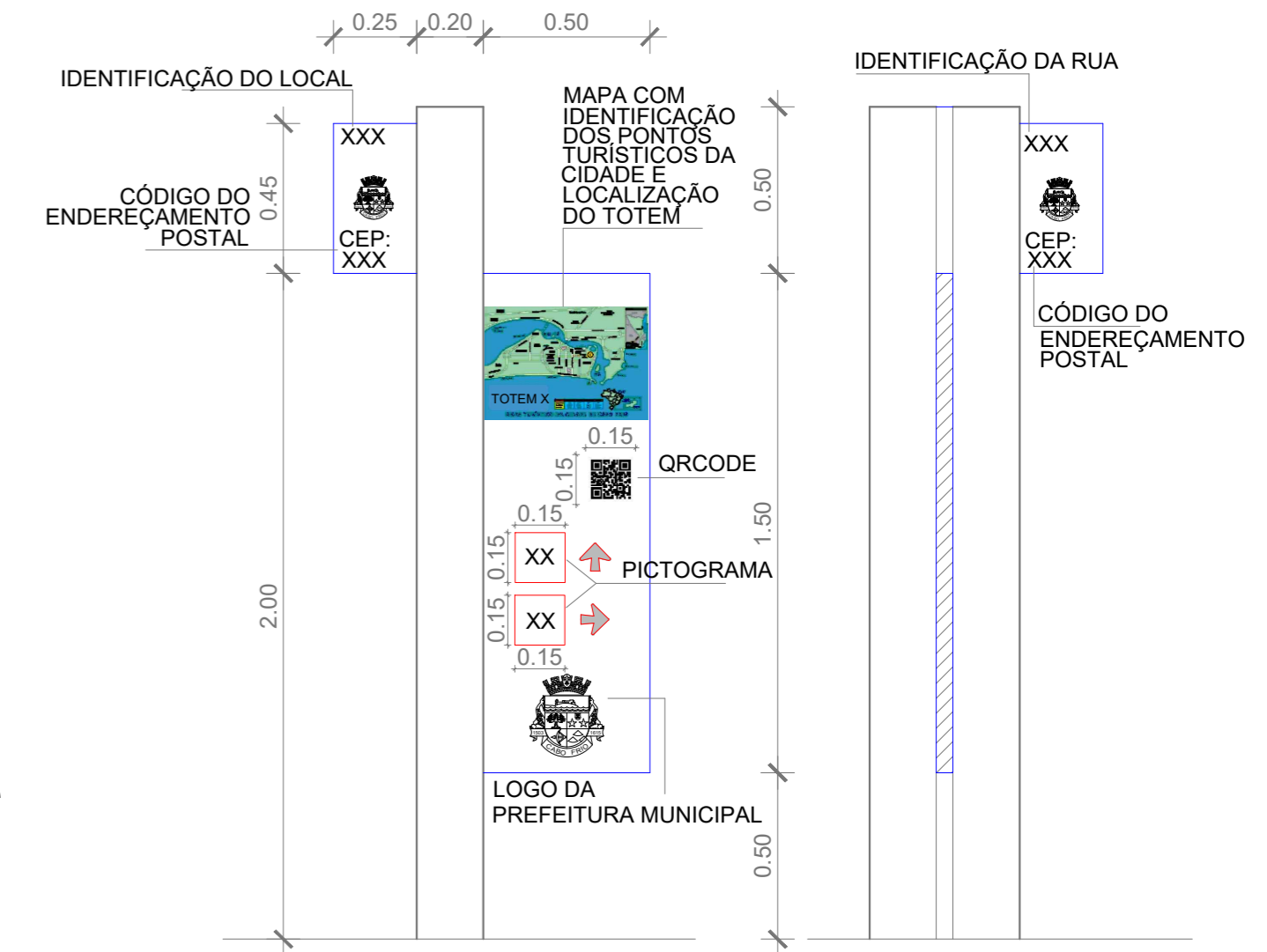
TOTENS DE SINALIZAÇÃO TURÍSTICA - DETALHE TÍPICO ESCALA: 1:20
