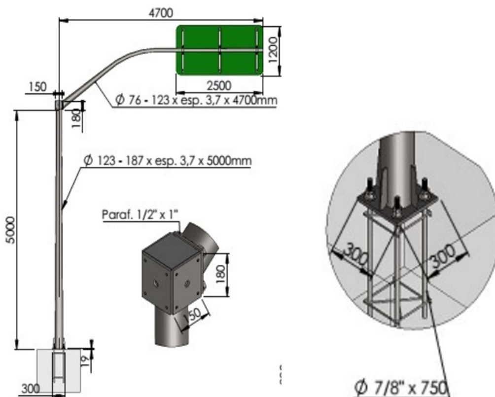
Figura 2 – Coluna cônica tipo I.
