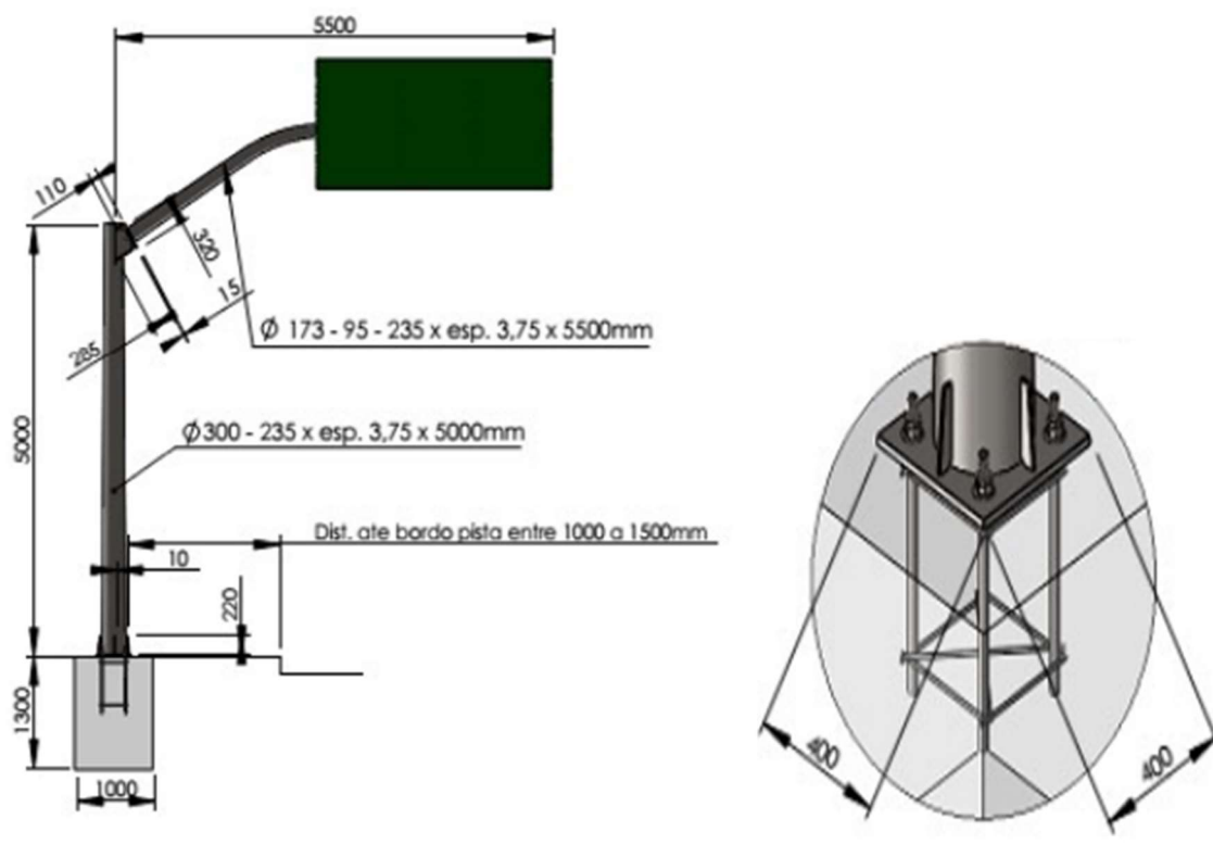
Figura 2 – Coluna cônica tipo II.
